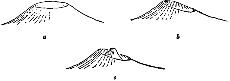
चित्र २०५—विसूवियस की ऐतिहासिक दशायें
